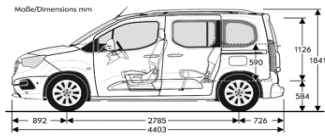
Maße/Dimensions mm
