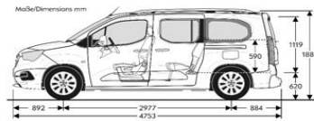
Maße/Dimensions mm
