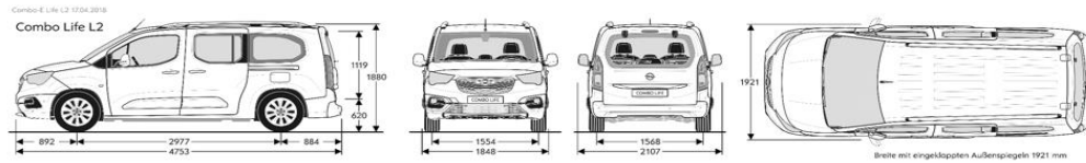
Maße/Dimensions mm
