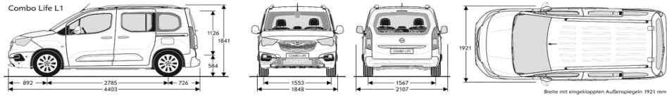
Maße/Dimensions mm
